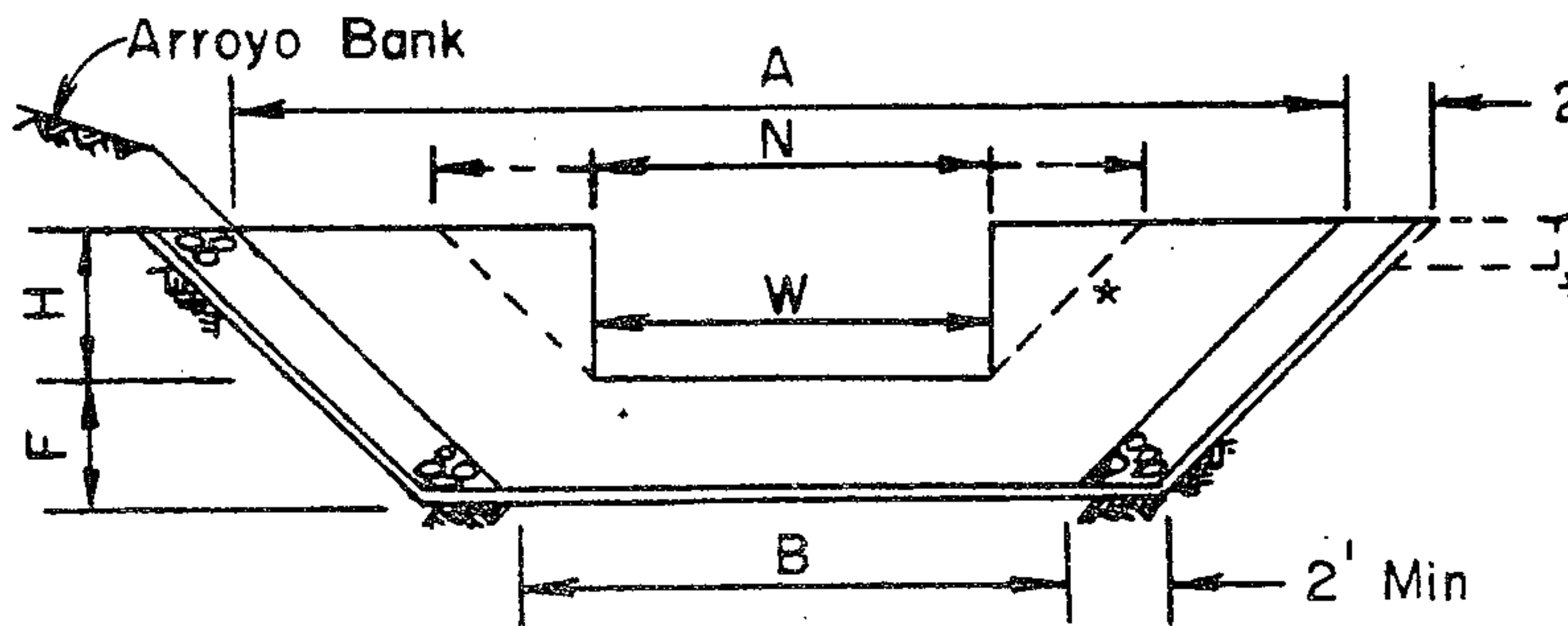
SECTION A-A
