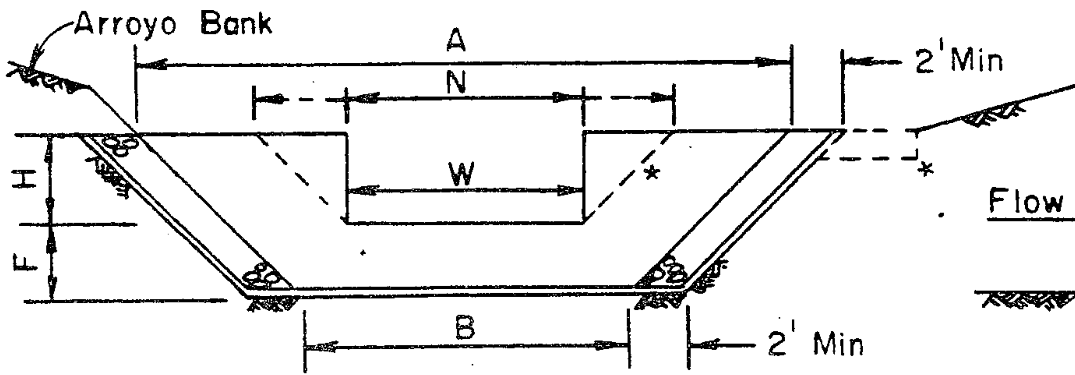
SECTION A-A
