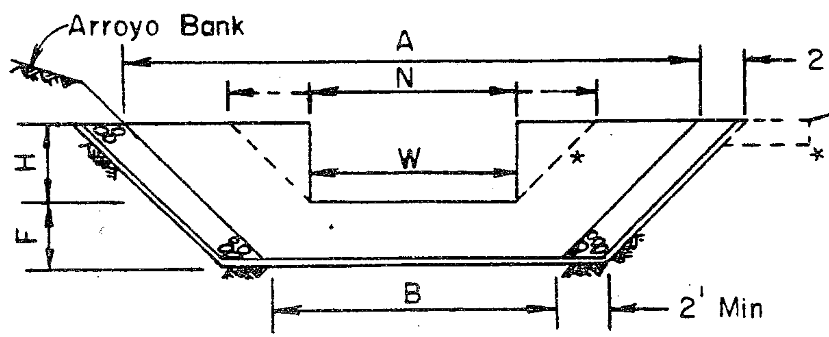
SECTION A-A
